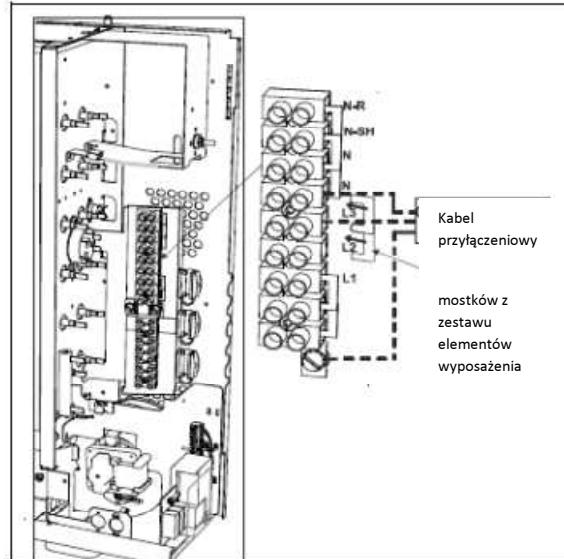
Rys. 29: Jednofazowe połączenie zasilania
