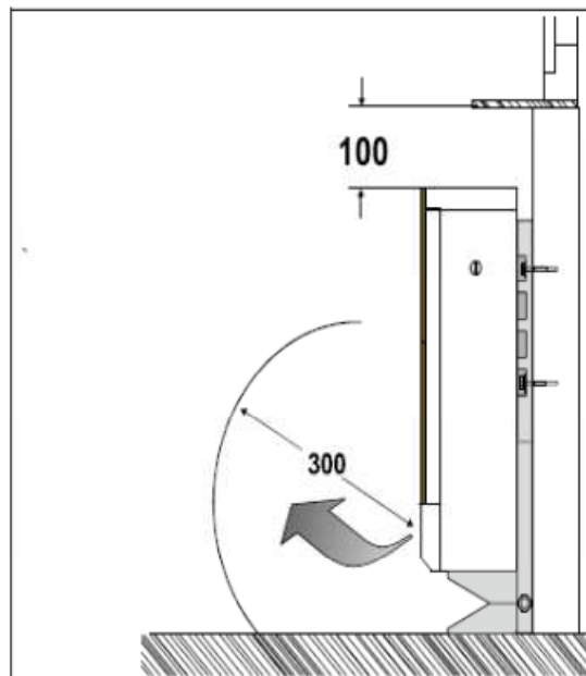
Rys. 8: Montaż ścienny/podłogowy przy użyciu wsporników WKO18.
