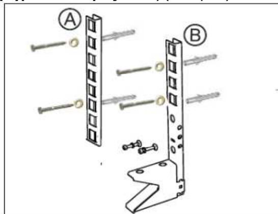
Rys. 5: Dostarczone wyposażenie: wspornik ścienny i wspornik ściennie/podłogowy WKO18
