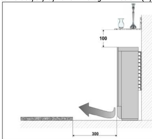
Rys. 4: Odległość od kratki wylotu powietrza.
