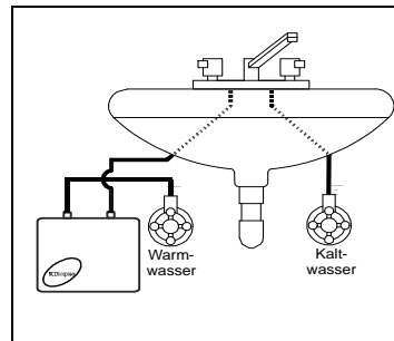
Abb. 4: Nacherwärmung
