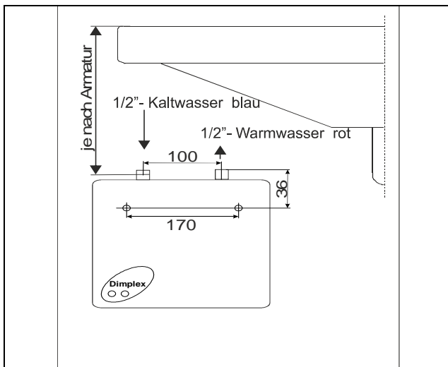
Abb. 2: Montage DZU 353
