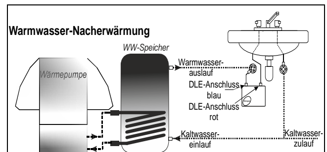
Abb. 5: Schema Warmwasser- Nacherwärmung
