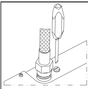
Abb. 6: Einstellen der Wasserdurchflussmenge
