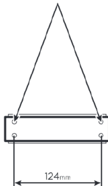
4 Otwory mocujące
